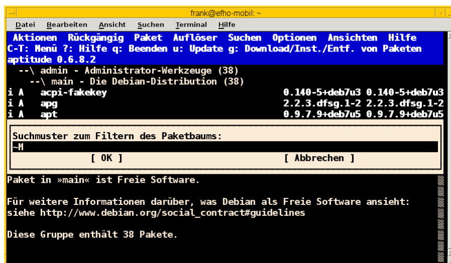
Abbildung 8.3: Ansicht der automatisch installierten Pakete in aptitude
