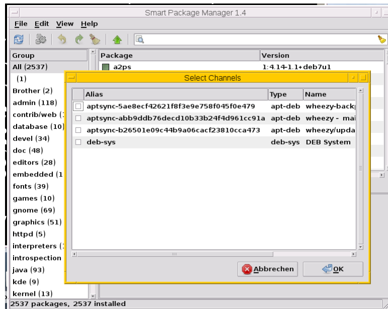
Abbildung 3.12: Auflistung der verfügbaren Paketquellen in SmartPM
