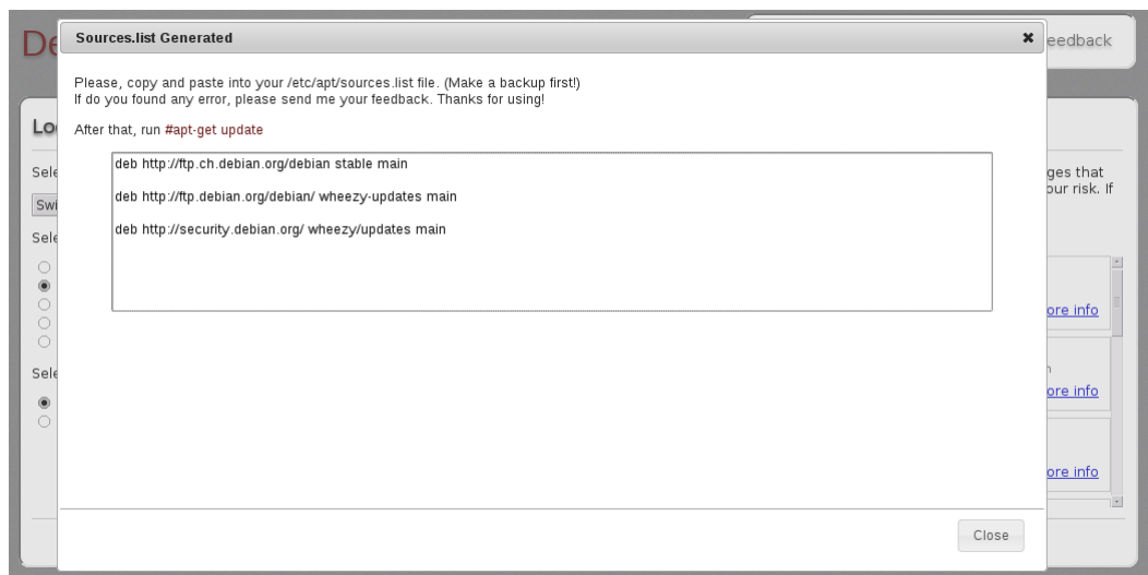
Abbildung 3.9: Erzeugte sources.list durch den Debian Sources List Generator
