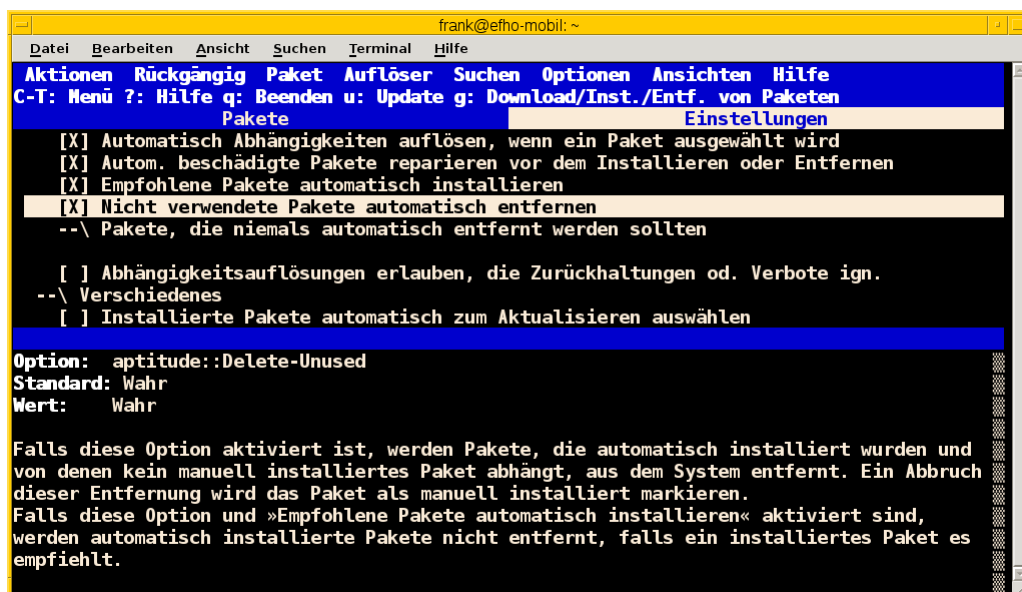
Abbildung 8.33: Nicht verwendete Pakete automatisch entfernen in aptitude
