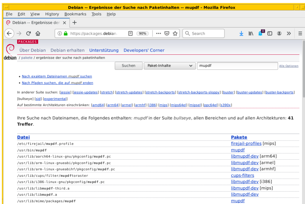
Abbildung 8.22: Suche nach der Zeichenkette mupdf über die Webseite des Debian-Projekts (Suchergebnis)
